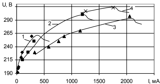
Рис.3. Зависимость напряжения от полного тока при отношениях радиусов электродов: 1 – 0,22; 2 – 0,36; 3 – 0,55; 4 – 0,73
