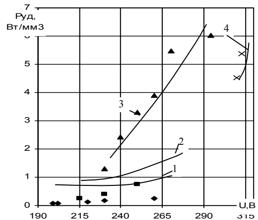
Рис.4. Зависимость удельных мощностей электродной системы от напряжения при отношении радиусов электродов: 1 – 0,22; 2 – 0,36; 3 – 0,55; 4 – 0,73
