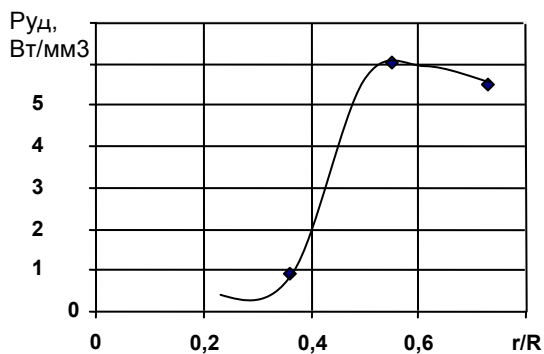
Рис. 6. Зависимость удельной мощности разряда P_{уд} , выделяемой в единице объема межэлектродного пространства полого катода, от отношения радиусов электродов r/R
