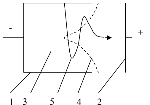
Рис. 1. Схематический рисунок, поясняющий эффект потенциальной ловушки. 1–полый катод; 2–анод; 3–межэлектродное пространство полого катода; 4–граница высокоионизированной плазмы; 5–траектория электрона, совершающего колебания внутри полого катода.
